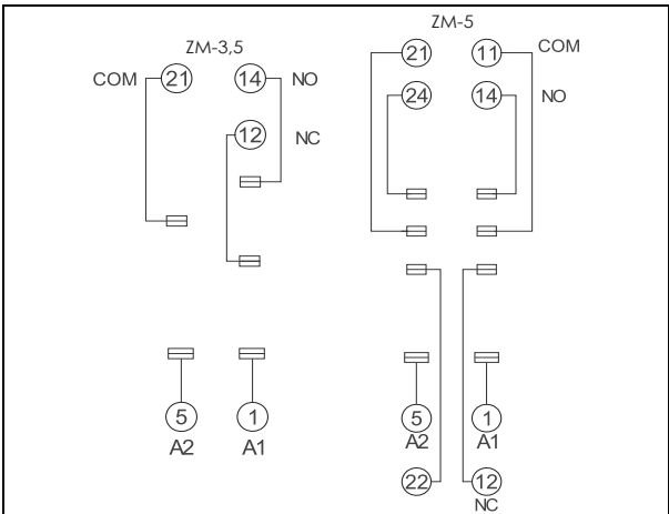
SCHEMA DI COLLEGAMENTO - WIRING DIAGRAM
