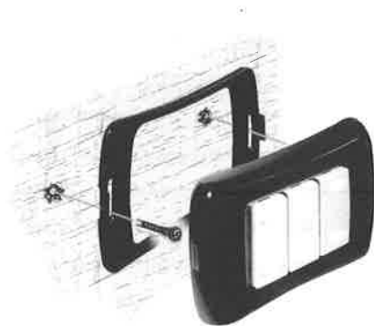
INSTALLAZIONE CON VITI SU PARETI RUSTICHE
