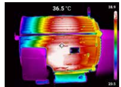
Immagine a infrarossi del motore dalla termocamera Fluke TiS75+
