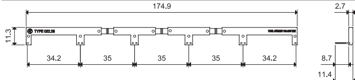
Pettine a 6 poli per tipi 22.34, larghezza 35 mm 022.26 (blu) Valori nominali 10 A - 250 V
