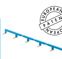
Pettine a 6 poli per tipi 22.34, larghezza 35 mm 022.26 (blu) Valori nominali 10 A - 250 V
