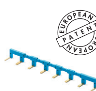
Pettine a 8 poli per tipi 22.32, larghezza 17.5 mm 022.18 (blu) Valori nominali 10 A - 250 V
