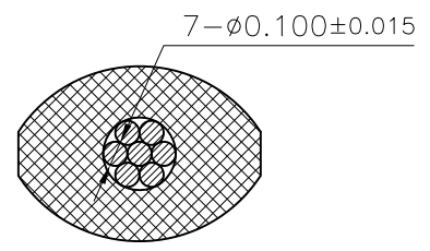
SECTION A-A (4:1)
